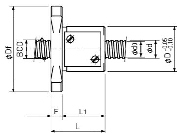
Type-1:Return-plate type リターンプレート式
