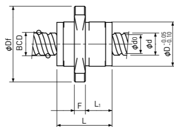
Type-3:End-cap type or End-deflector type エンドキャップ式またはエンドデフレクタ式
