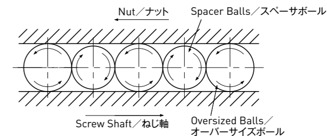
図 A-106 : スペーサボール Fig. A-106 : Spacer Balls
