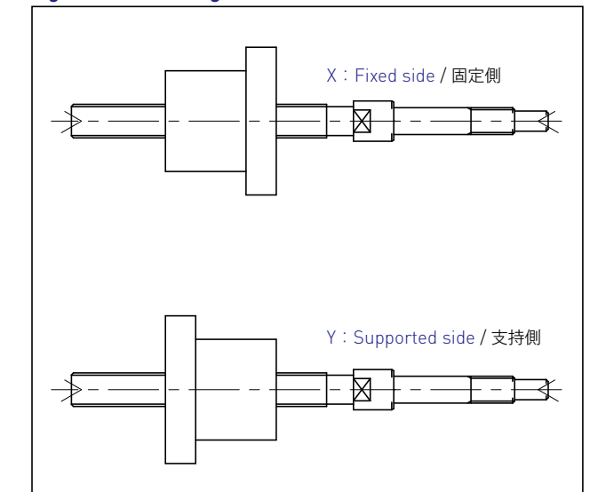
図 A-2：ナットフランジ向き Fig. A-2：Nut Flange direction
